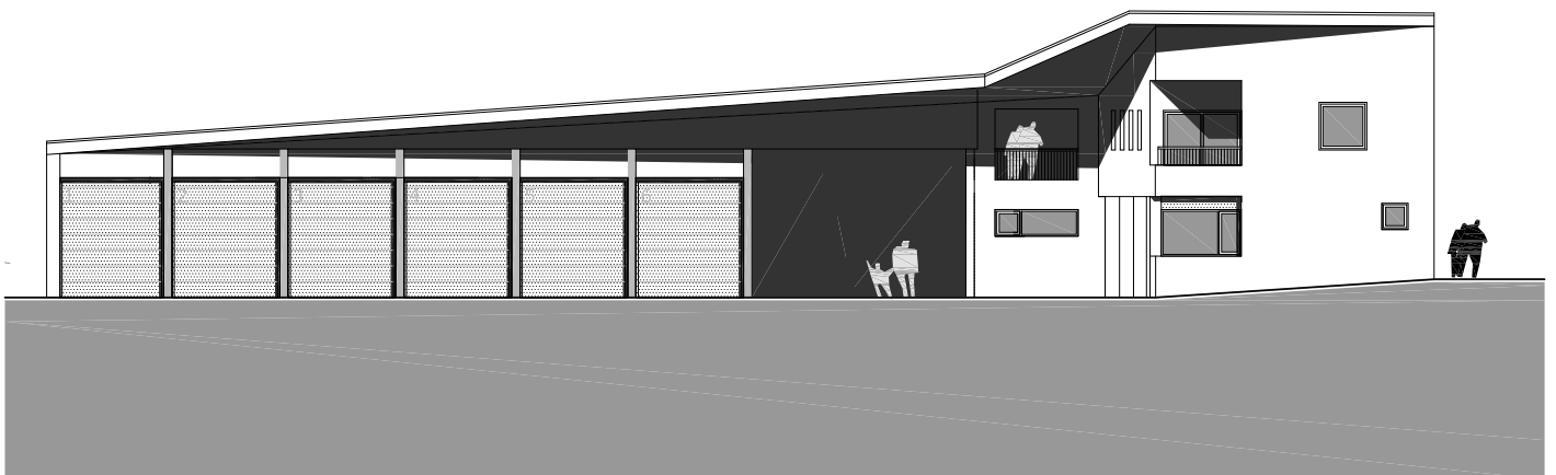
Ansicht Süd
