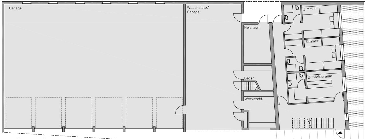
Erdgeschoss
